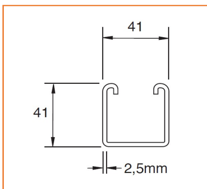
Vista Lateral
